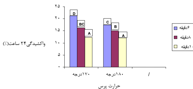
شکل ۲۴- اثرگذاری متقابل زمان پرس و دمای پرس بر واکسیدگی ضخامت (۲۴ ساعت) و گروه‌بندی
